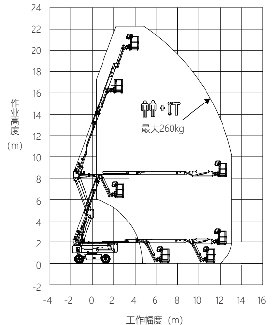
LA20JE性能曲线图
